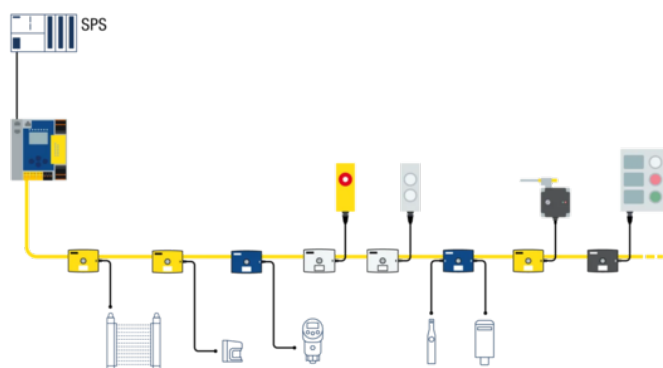
Fig.: i distributori attivi e passivi possono essere montati facilmente lungo il cavo ASi.
