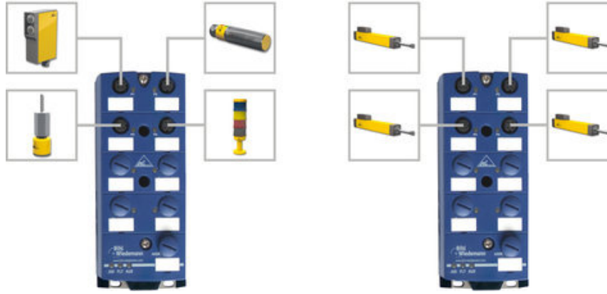
Fig.: AS-i/IO-Link Modülleri, I/O-Link Kontrolör -4 IO-Link Port Class A ( BWU2853 ) veya Class B ( BWU3020 ) - birçok üreticinin IO-Link ürünleri ile mükemmel uyumluluk
