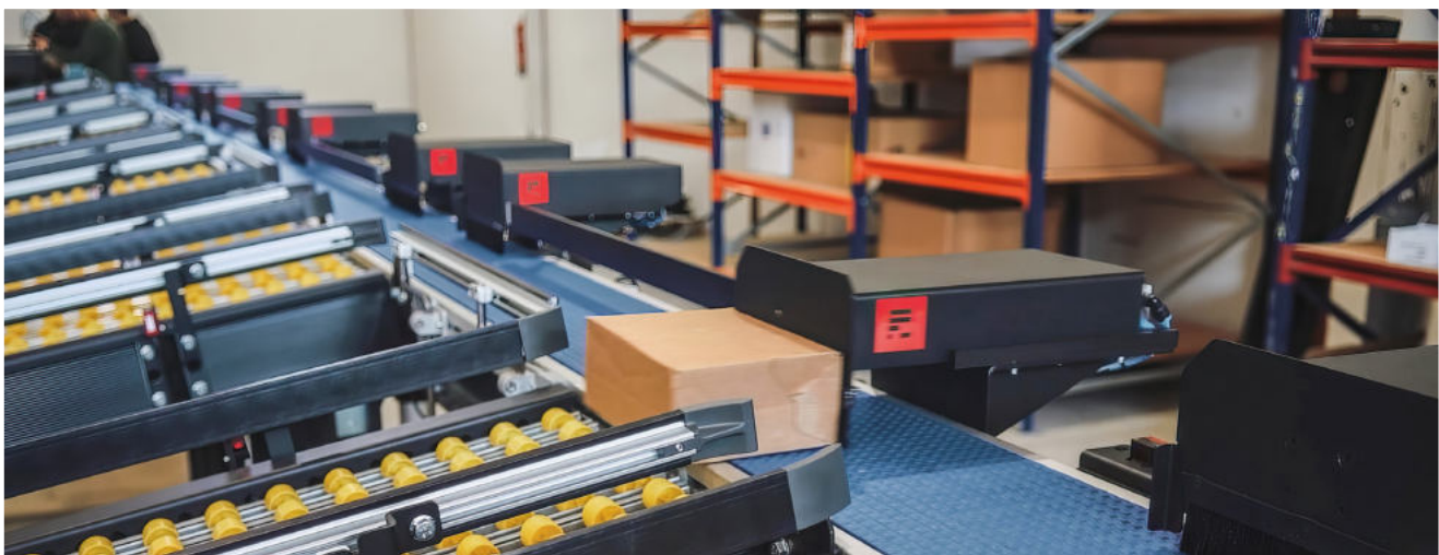
Ausschleusung eines Pakets mit Hilfe pneumatischer Aktuatoren
