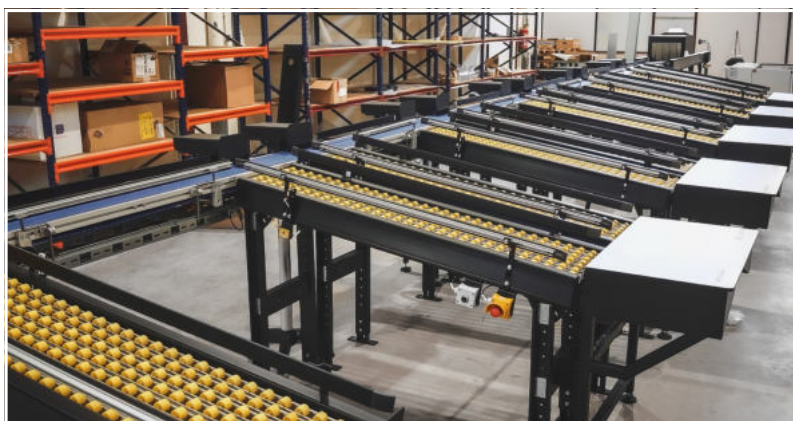
Mit dem RIELEC Fit Sorter Paketsortierer lassen sich bis zu 1800 Kartons in einer Stunde sortieren.
