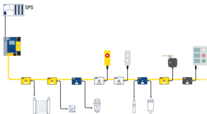
Fig.: Aktive og passive distributører kan nemt monteres langs ASi-kablet.
