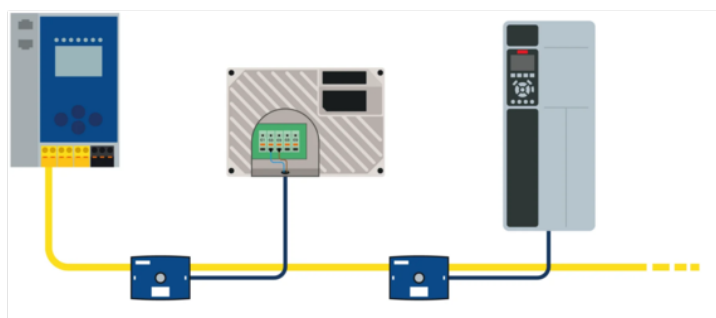
Fig.: Los distribuidores activos y los distribuidores pasivos se pueden montar fácilmente a lo largo de la línea ASi.
