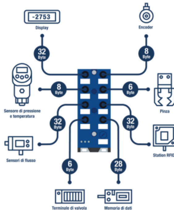
Fig.: Il nuovo master IO-Link a 8 porte ( BWU4386 ) è la soluzione più conveniente di Bihl+Wiedemann per singola porta, grazie anche alla facile tecnologia di collegamento ASi.
