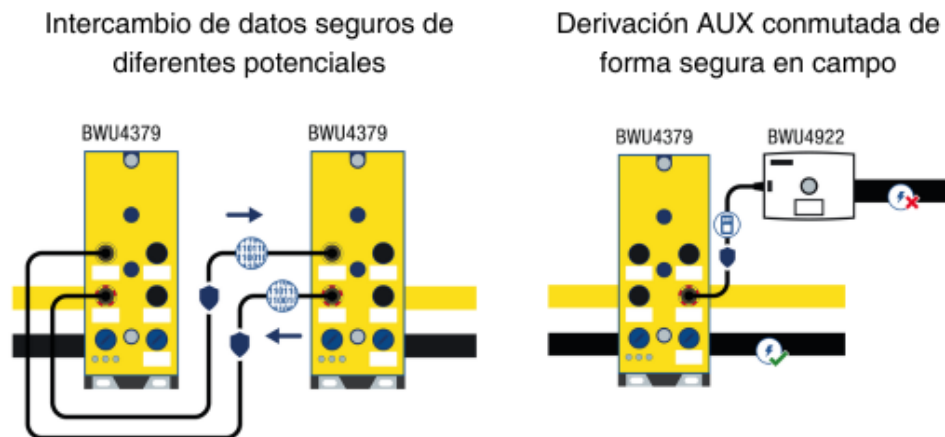
Fig.: Intercambio de datos seguros entre dos partes de la instalación con diferentes circuitos ASi y potenciales AUX con dos cables M12 estándar ( izquierda ). Generación de una derivación AUX conmutada de forma segura con ayuda de un distribuidor pasivo para desconectar de forma pasiva segura varios participantes ( derecha ).
