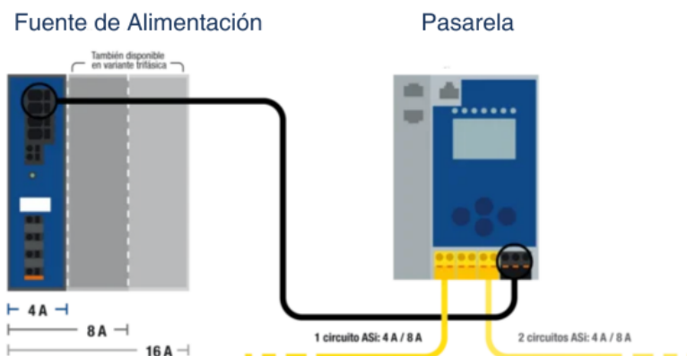
Fig.: Las fuentes de alimentación de 30 V son significativamente más compactas en comparación con las fuentes de alimentación ASi con bobinas de desacoplamiento. Además, ya que se pueden poner en fila, ahorran mucho espacio en el armario eléctrico.
