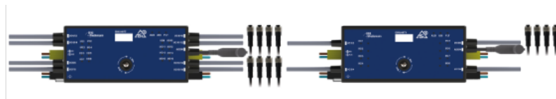
Fig.: Los módulos E/S auto-configurables para el canal porta-cables son el complemento perfecto para su tecnología para manutención. Están disponibles con 16 E/S (BWU4977) y 8 E/S (BWU4979).
