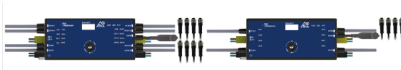
Fig.: I moduli I/O autoconfigurabili per canalina sono il completamento ideale per il vostro sistema di movimentazione dei materiali. Sono disponibili con 16 I/O ( BWU4977 ) e 8 I/O ( BWU4979 ).
