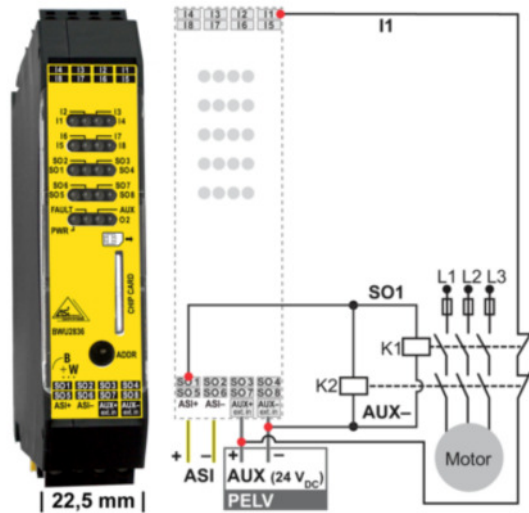
Abb.: Das neue AS-i Safety Ausgangsmodul mit 8 sicheren Ausgängen (BWU2836)
