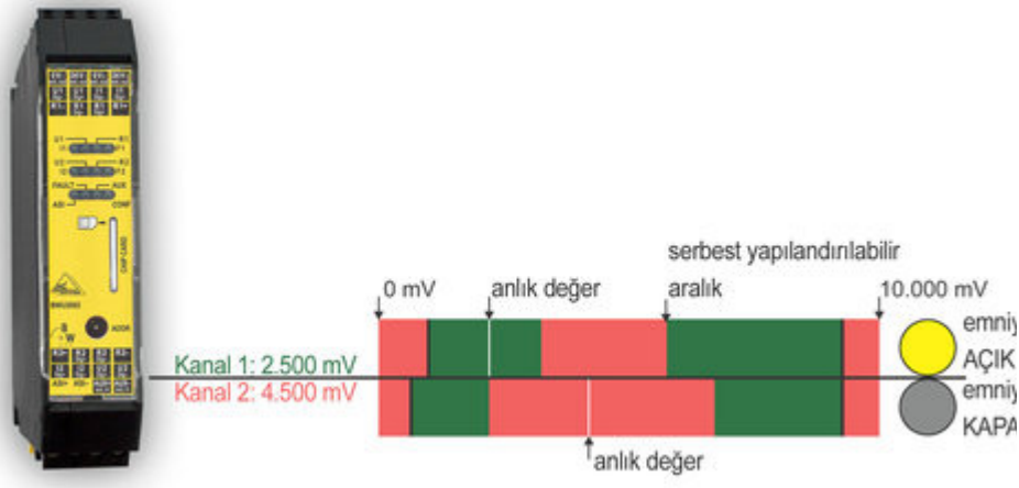
Fig.: Yeni AS-i Emniyet Analog Giriş Modülü (BWU2692)
