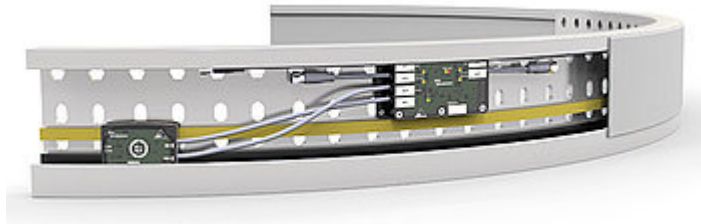
Fig. 2: Modulo per motorullo (BW3278, BW3290) nella canalina
