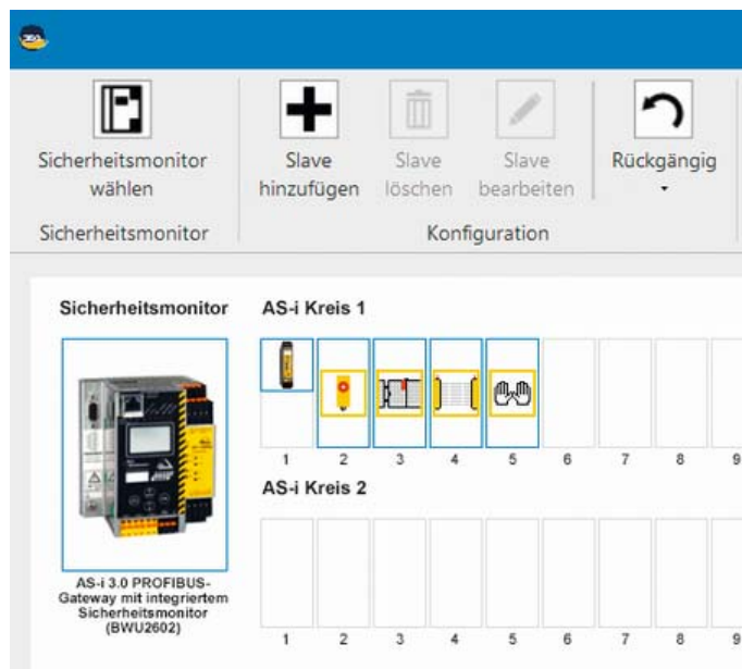
Abb. 2: Einfache Hardwarekonfiguration mit ASIMON360
