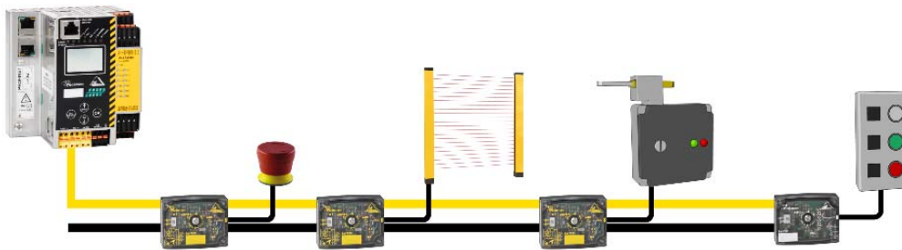
Fig. 2 : Répartiteurs actifs : tout type de capteurs et actionneurs peut communiquer via AS-i
