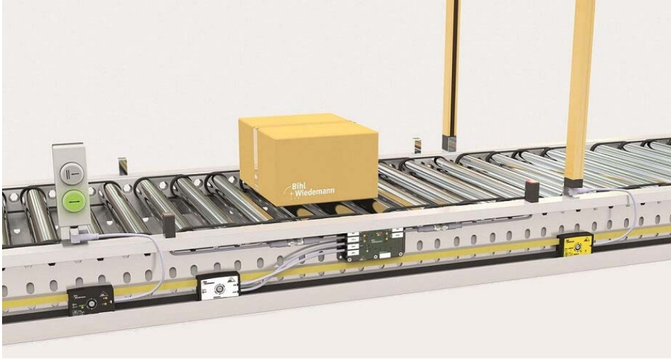
Fig. 1: Utilizzare i distributori attivi per rendere qualsiasi componente compatibile con il bus
